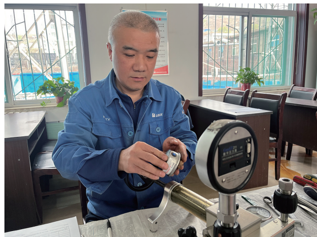
洗煤厂于今年承接了汾西矿业在用压力表周期检定工作。检定人员严格按照检定规程,对压力表的外观、示值误差、轻敲位移、回程误差以及指针偏转的平稳性等因素进行检定。对检定合格的压力表,检定人员加贴绿色合格标签,并出具检定证书。今年以来,洗煤厂已为双柳煤矿、贺西煤矿等20家单位完成5000余块压力表的检定。 刘媛 摄影报道
